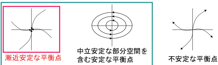
Lyapunov 安定な平衡点
